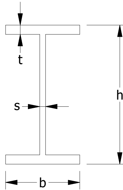
IPE
