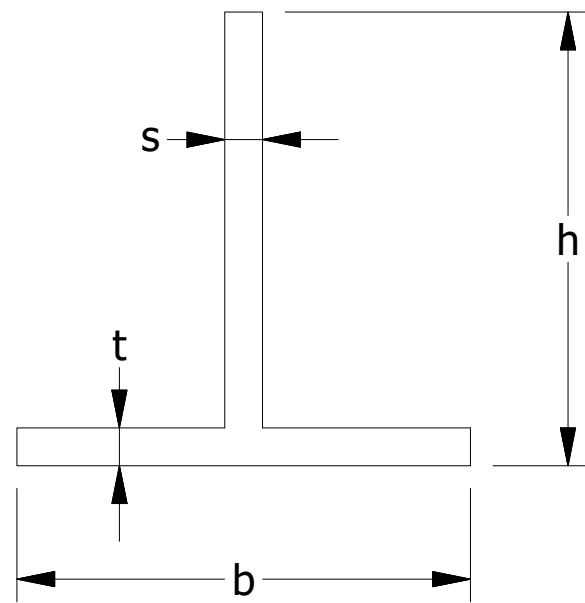
T-Profile
